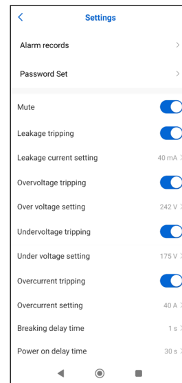
Configuración protecciones
